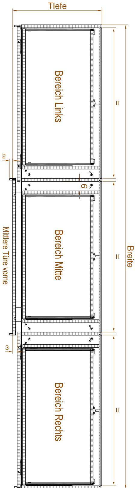
Schnitt A-A
