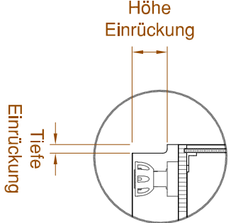
Sockeleinrückung hinten:
