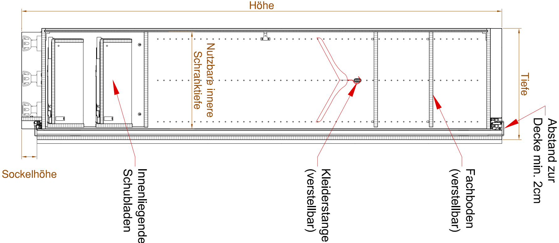
Schnitt B-B
